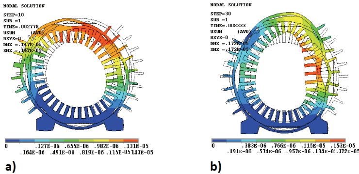
Rys. 4. Postać deformacji U[m] stojana dla silnika z ekscentrycznością statyczną dla wybranych położen wirnika: a) 10 stopni; b) 30 stopni
