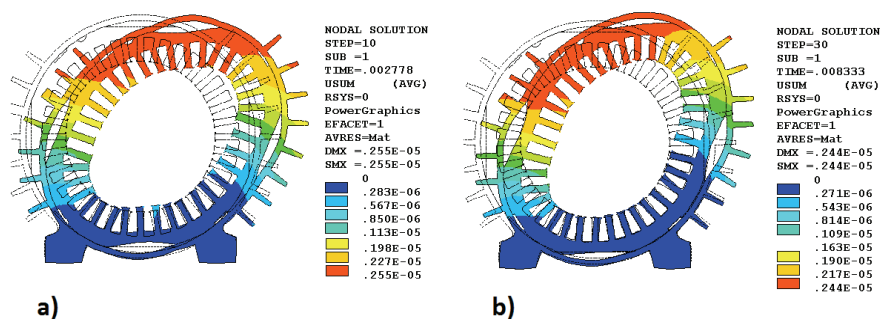
Rys. 8. Postać deformacji U [m] stojana dla modelu B dla wybranych położeń wirnika: a) 10 stopni; b) 30 stopni Fig. 8. Shape of deformation of stator structure U [m] for model B for selected positions of rotor: a) 10 degree; b) 30 degree
