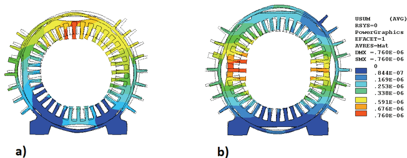
Rys. 3. Postać deformacji U [m] stojana dla silnika o idealnym centrycznym położeniu wirnika i symetrycznym poziomie namagnesowania magnesów dla wybranych położeń wirnika:
