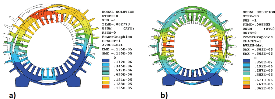
Rys. 7. Postać deformacji U [m] stojana dla modelu A dla wybranych położeń wirnika: a) o 10 stopień; b) 30 stopni Fig. 7. Shape of deformation of stator U [m] for model A for selected positions of rotor: a) 10 degree; b) 30 degree
