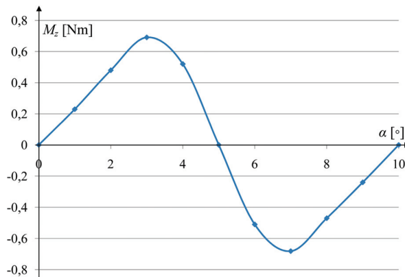
Rys. 6. Moment zaczeowy M_z = f(\alpha)
