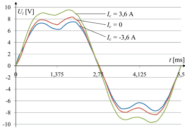
Rys. 5. Napięcie indukowane U_i = f(t) dla n = 30 obr/s
