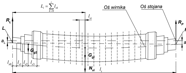
Rys. 4. Wirnik podzielony na elementy tarczowe Fig. 4. Rotor divided into disc elements
