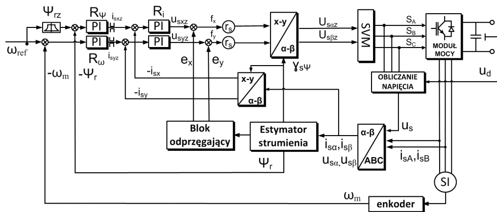
Rys. 1. Struktura układu sterowania połowo zorientowanego dla napędu z silnikiem indukcyjnym
